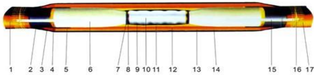
1 铜屏蔽带 2 外半导电层 3、密封胶 4、应力疏散胶 5、应力控制管 6、XPLPE绝缘 7 内半导电层 8 导体 9、半导电带 10、连接管 11 填充胶 12 内绝缘管 13、外绝缘管 14、半导管 15、铜编织网 16 扎线 17 铜屏蔽网
